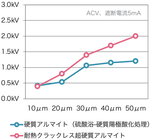
▼膜厚毎の絶縁破壊電圧
