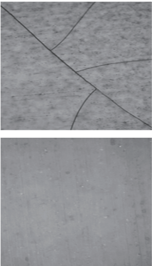
▼ 350℃熱処理後の一般アルマイト(上)とTAF TR(下)
