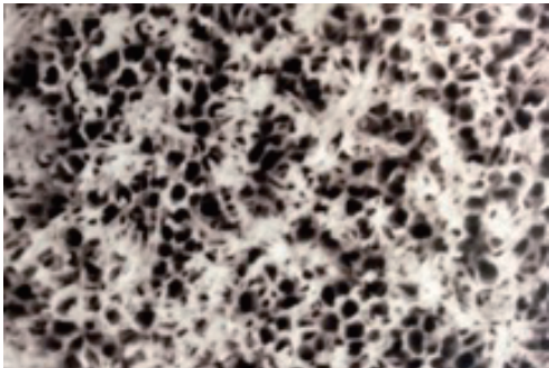
接着接合下地アルマイト表面電子顕微鏡写真
